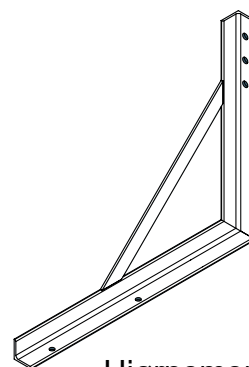
Hjørnemontert. Varmgalvanisert 125 kg.*
