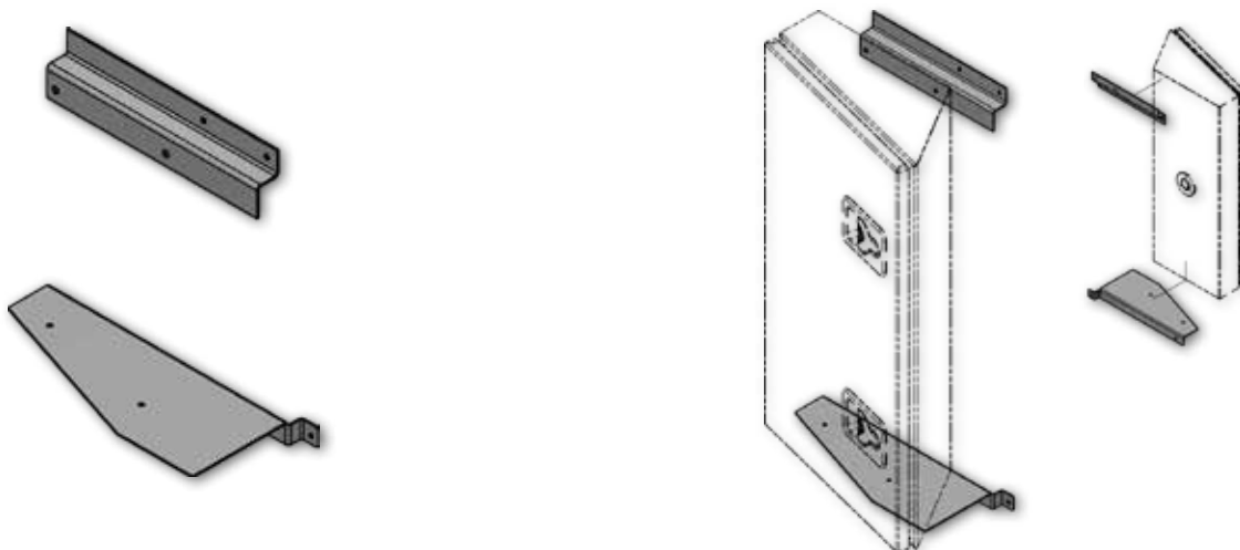
BRAKETT BevoBox™ høyre
