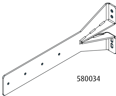
Type Y: Rett - forsterket. Varmgalvanisert 150 kg.*
