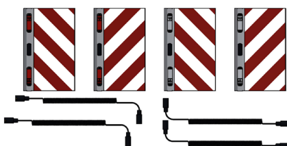
2005319 Breddmarkering m. ljus. Godk. SE/EU/NO 280x560 Set
